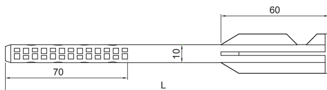
PREDNJI PRIKAZ
