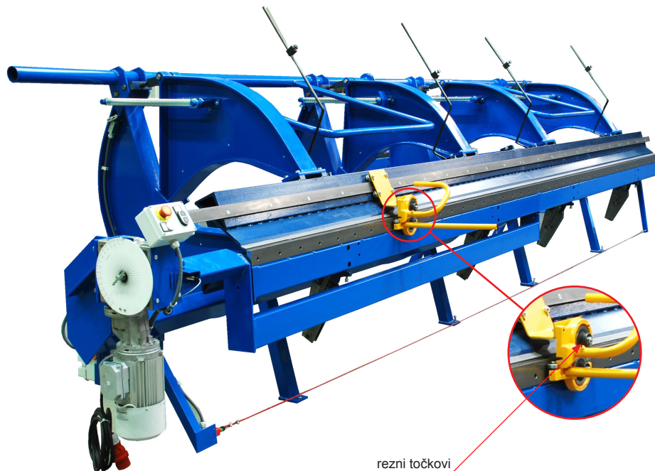
rezní točkovi
